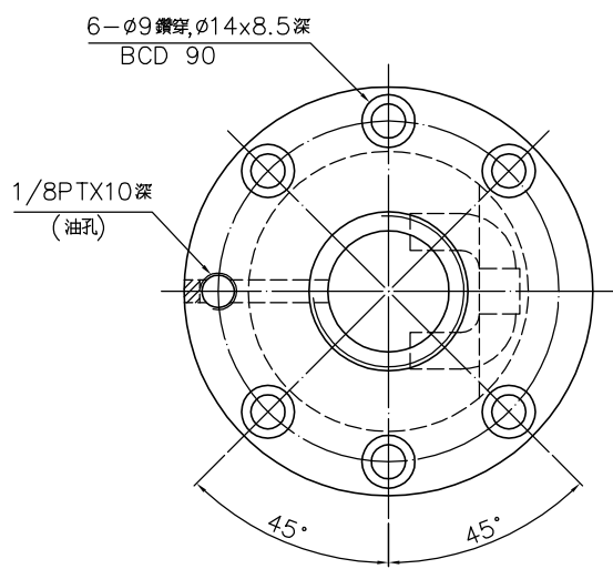
D-D 視圖
