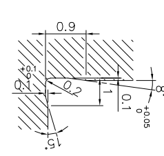
X 詳圖
